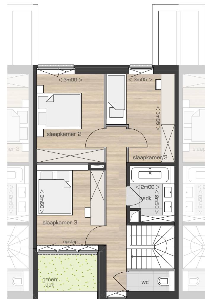
VERDIEPING
