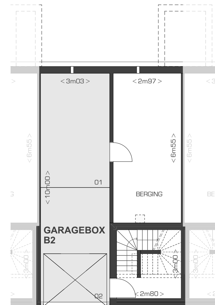
VERDIEPING
